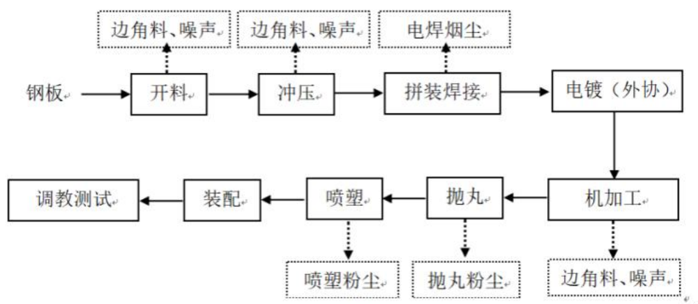
图 1 - 生产工艺及产污流程图。
