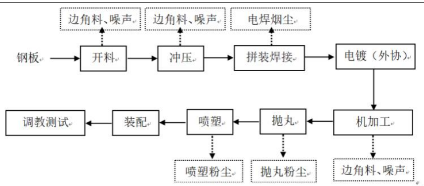
图1 生产工艺及产污流程图
